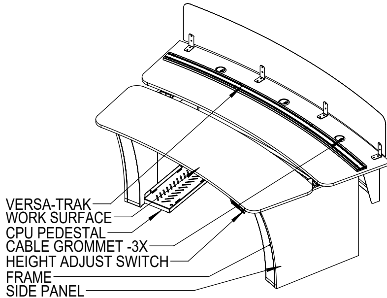
① Vue P Open Base Dual Sit-Stand ISO-Front
