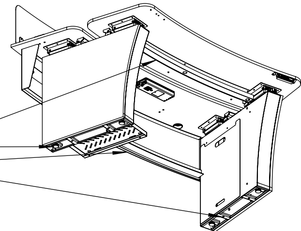
③ Vue P Open Base Dual Sit-Stand ISO-Bottom
